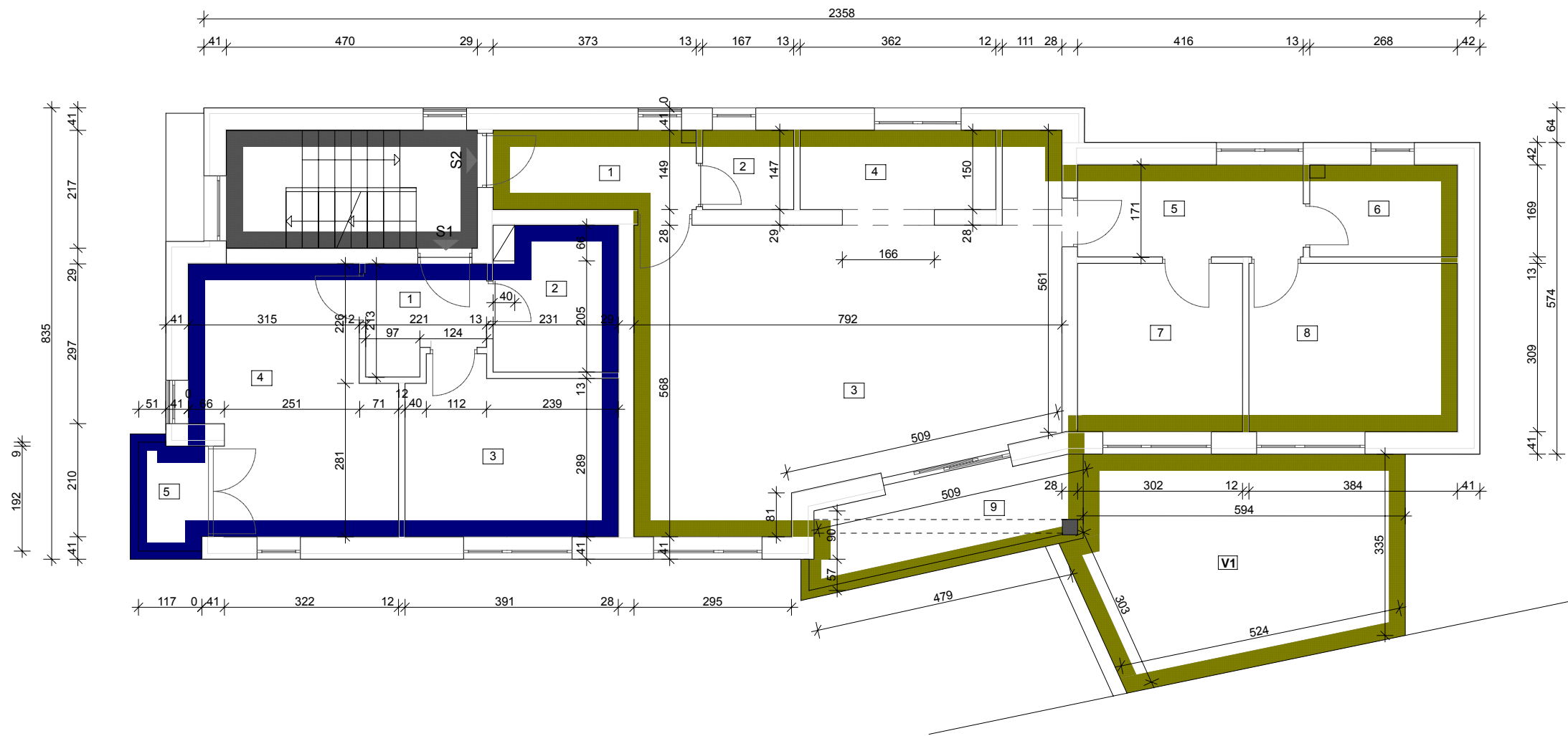
T L O C R T P R I Z E M L J A 1 : 100
